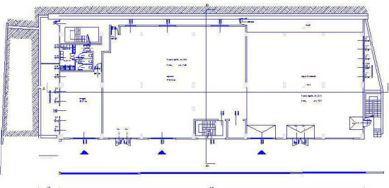
PIANTA PIANO SEMITERRATO
